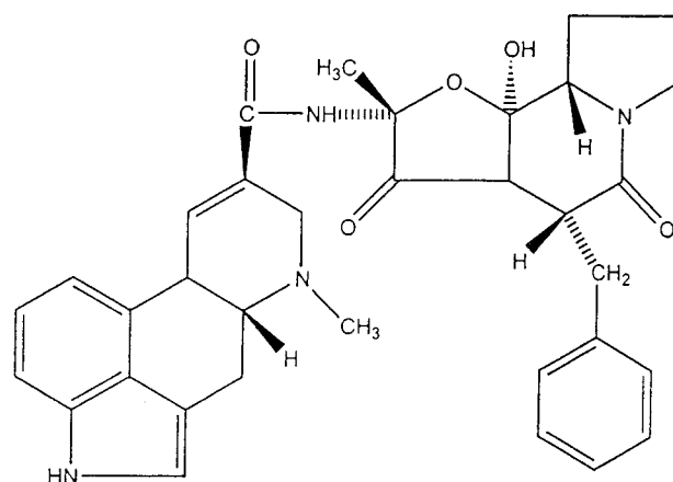
FIG. 3. Ergotamine.
