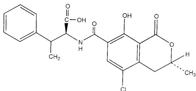
FIG. 5. Ochratoxin A.
